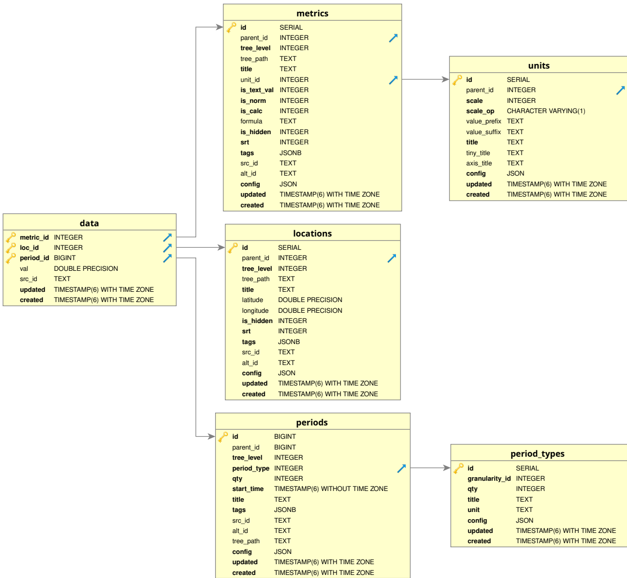
Рис. 1.1 Упрощенная схема данных LuxmsBI
